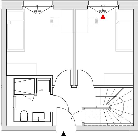
2. Obergeschoss
