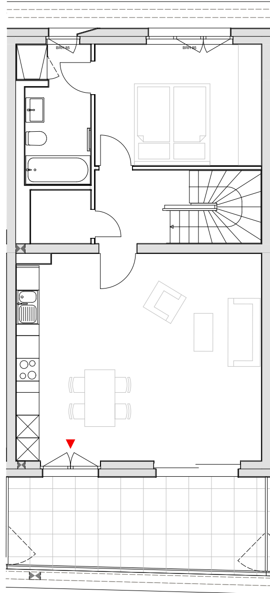
3.Obergeschoss/STG
