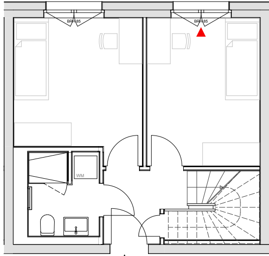
2.Obergeschoss
